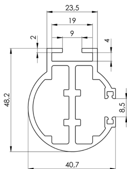
Kruhová vodicí lišta jednoduchá P 018/7 (7-302154)
