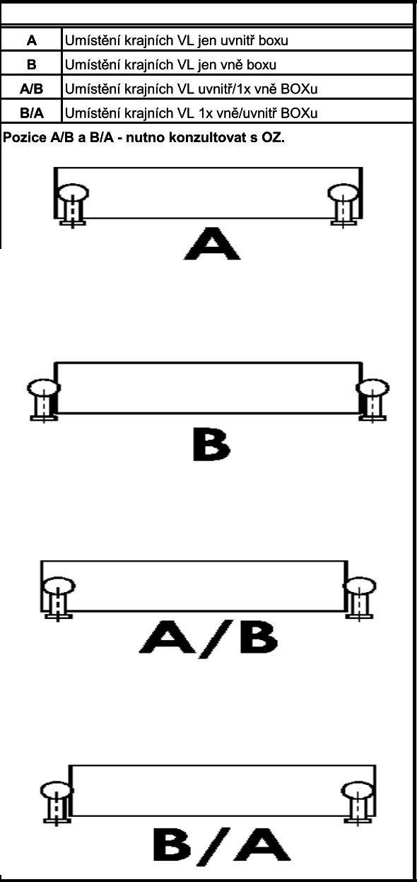
Provedení boxu a vodicích lišt
