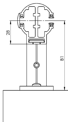
Upevnění vodicí lišty
