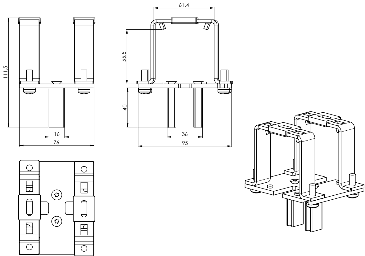
Patka dvojité Al P 002/9 (2-01628) pro STS P 016/2
