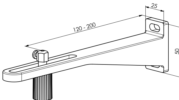
Vodítko lanka jednoduché, 120 - 200 mm P032/5 (2-01645)
