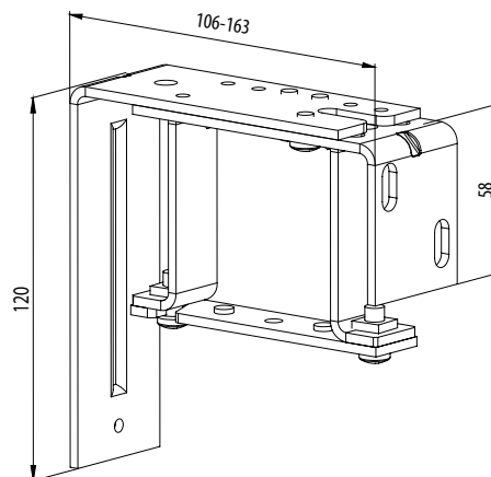
Držák nastavitelný (vnitřní věšák Al) 106-163 mm P 011/1 (2-00373) (pro horní profil 58 x 60)
