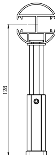
DRŽÁK VODÍCÍ LIŠTY P 021/6 2-00583-XXXX-0
