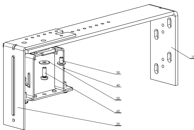
Držák nastavitelný dvojité – pevný 306 – 368 mm P 010/47 (2-01805-0000)
