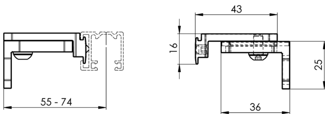
Držák vodící lišty 055 – 074 mm Zn P021/50 (2-01818-PU11)
