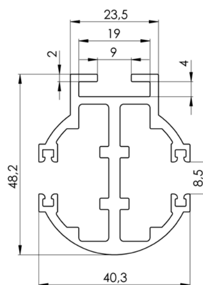
Kruhová vodicí lišta dvojitá P 017/7 (7-302155)
